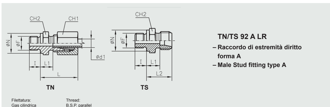
Forma A DIN 3852 Foglio 2
